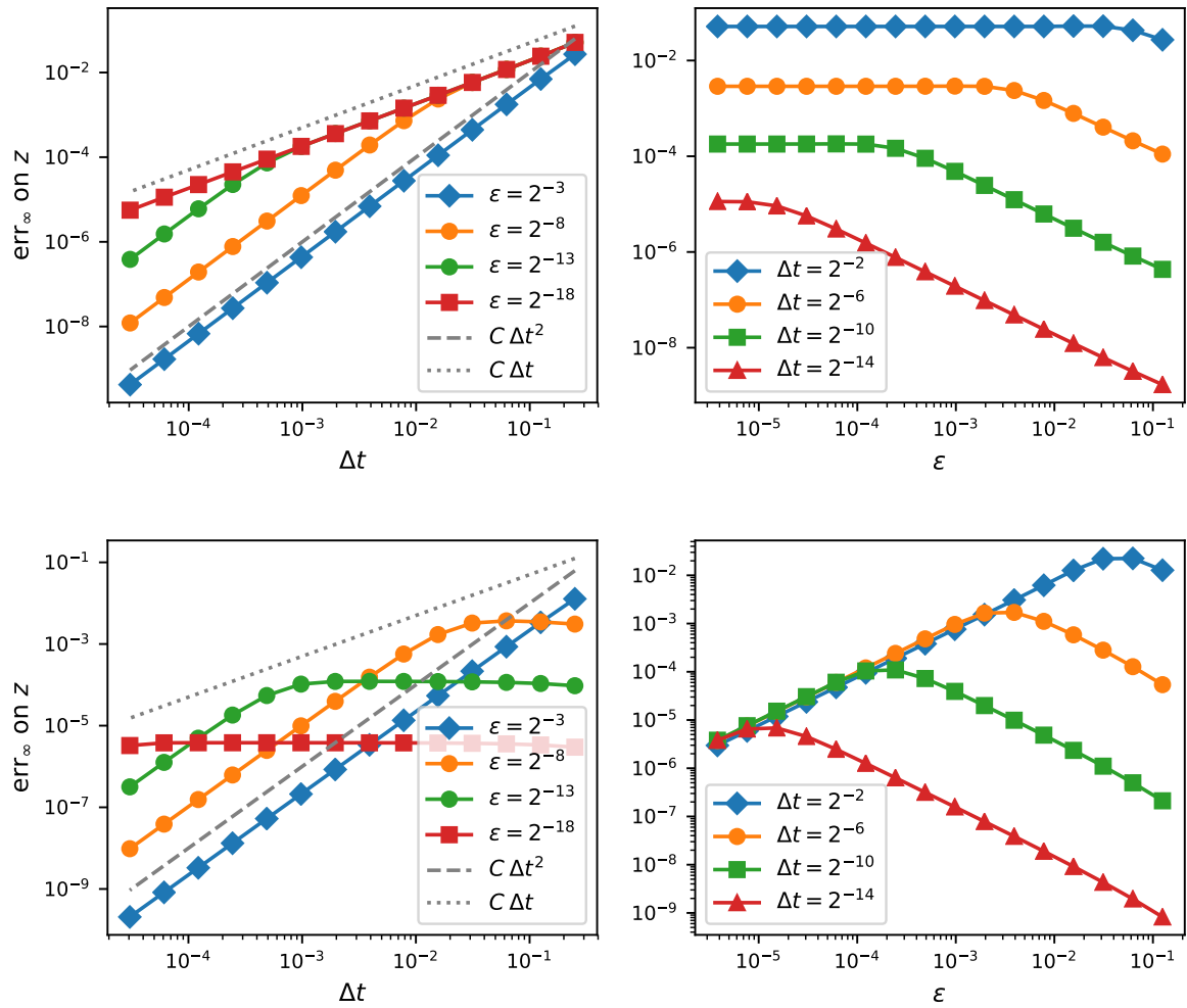
FIGURE 3 – Erreurs sur x (en haut) et z (en bas) en fonction de \Delta t (à gauche) et de \varepsilon (à droite) avec la méthode de Strang. Sur les tracés de l'erreur en fonction de \Delta t , les convergences théorique et uniforme sont tracées.
